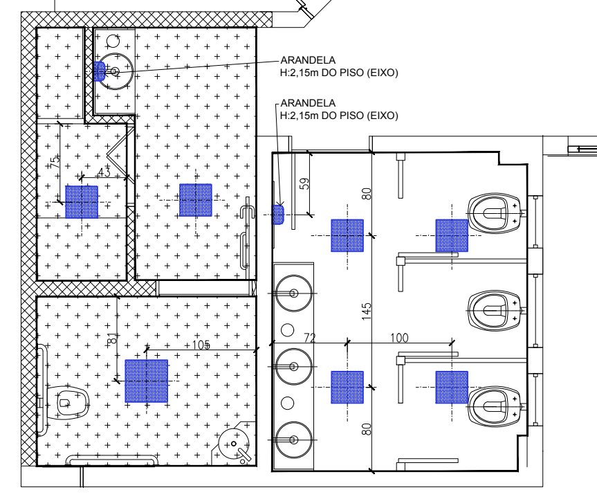
PLANTA FORRO/ILUMINAÇÃO Escala 1:50
